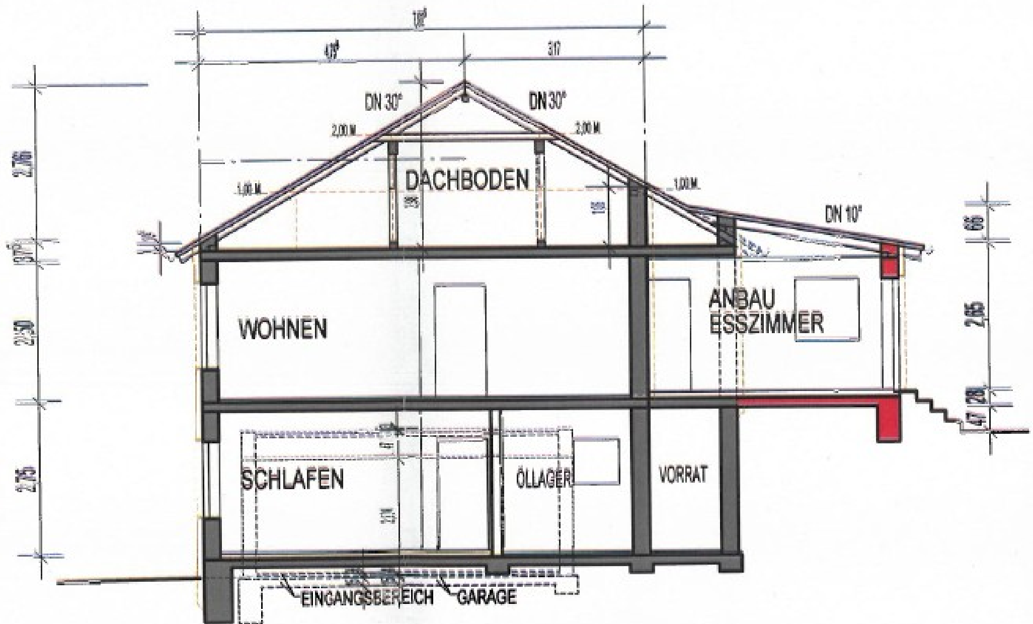
QUERSCHNITT: A.-B.
